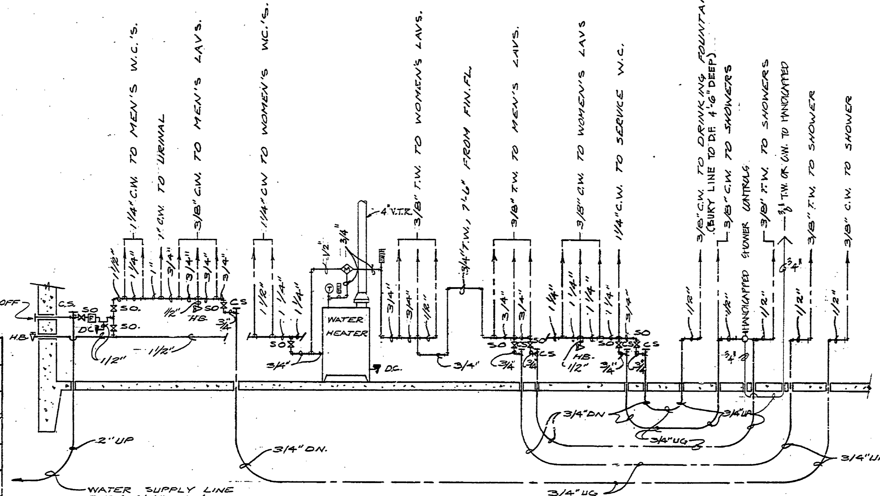
WATER RISER DIAGRAM N.T.S.
