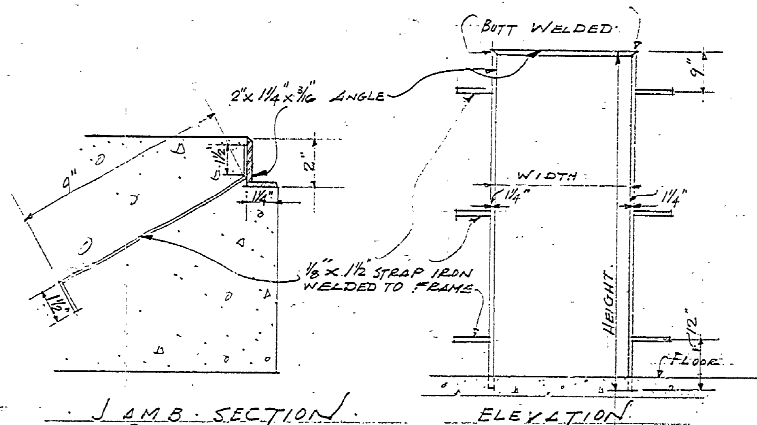
ELEVATION
