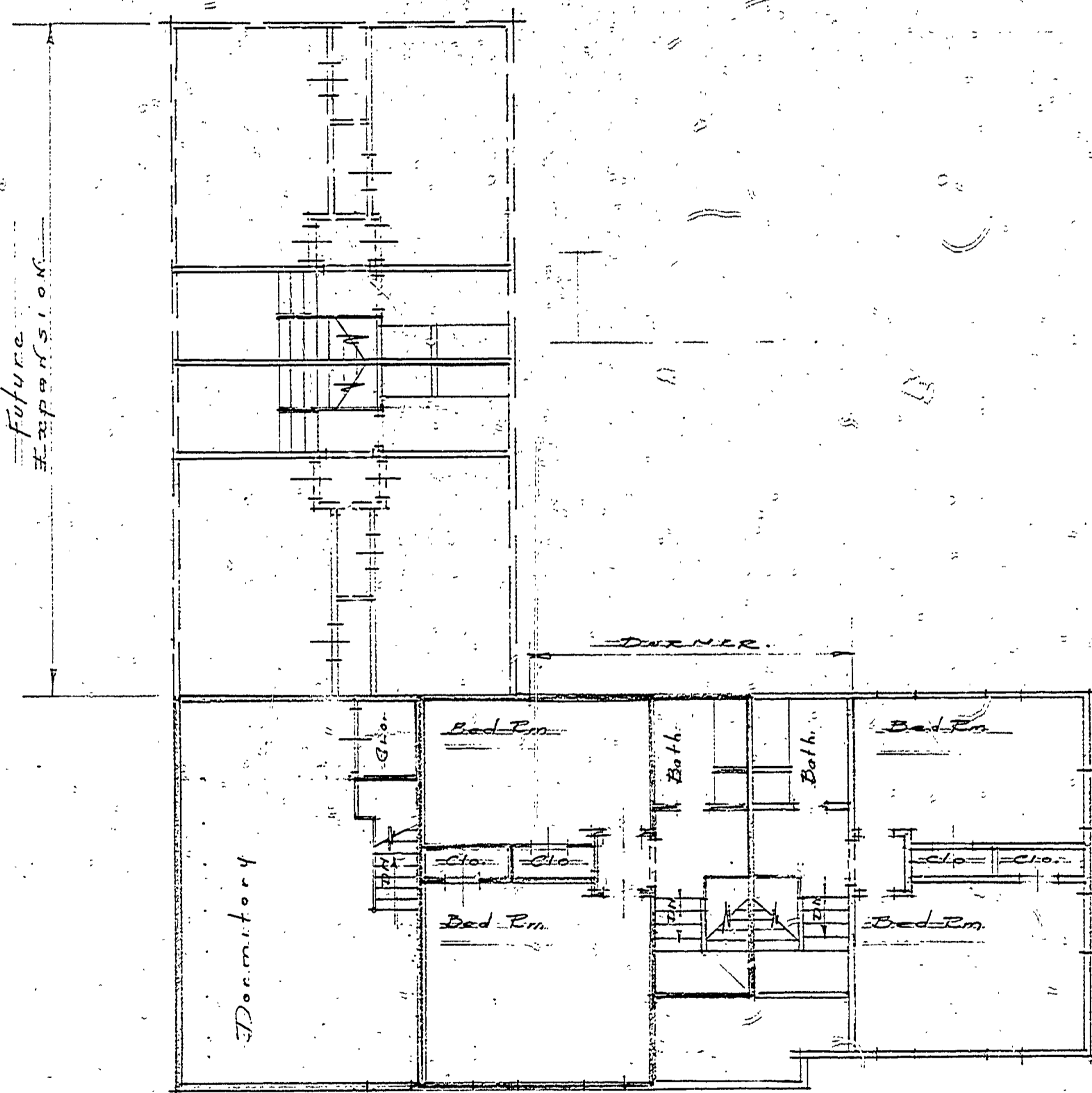
3-2-0-0-0 FLOOR PLAN 3-2-0-0-0
