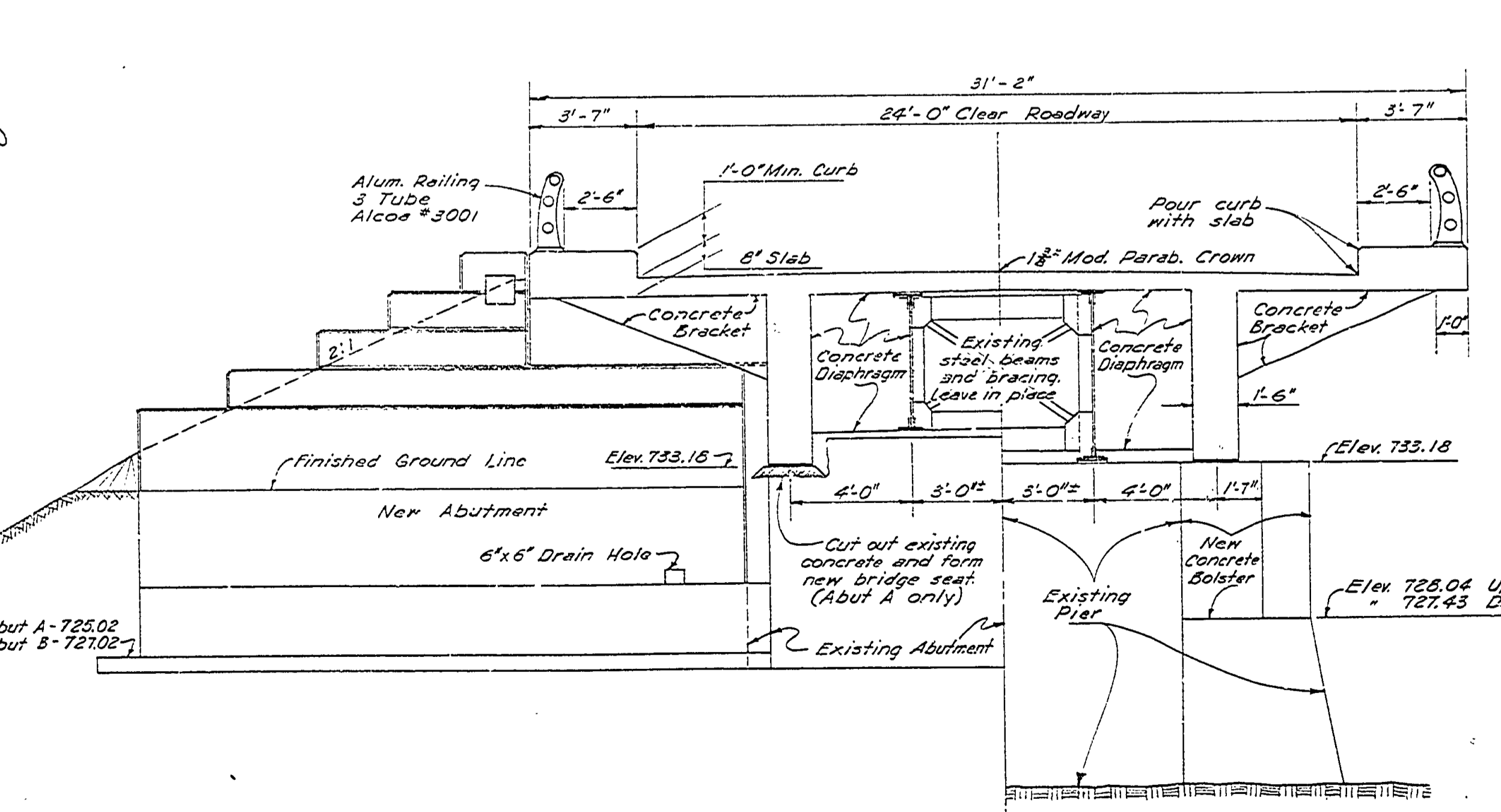
SECTION A-A 1/4"=1'-0"
