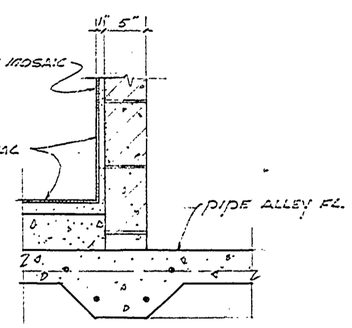
DET. @ FLOOR 16 2/4
