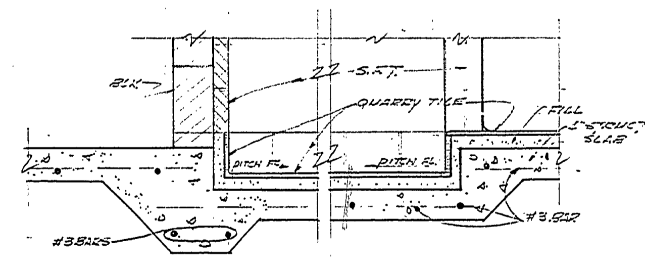
FL. DET. 18 2/4
