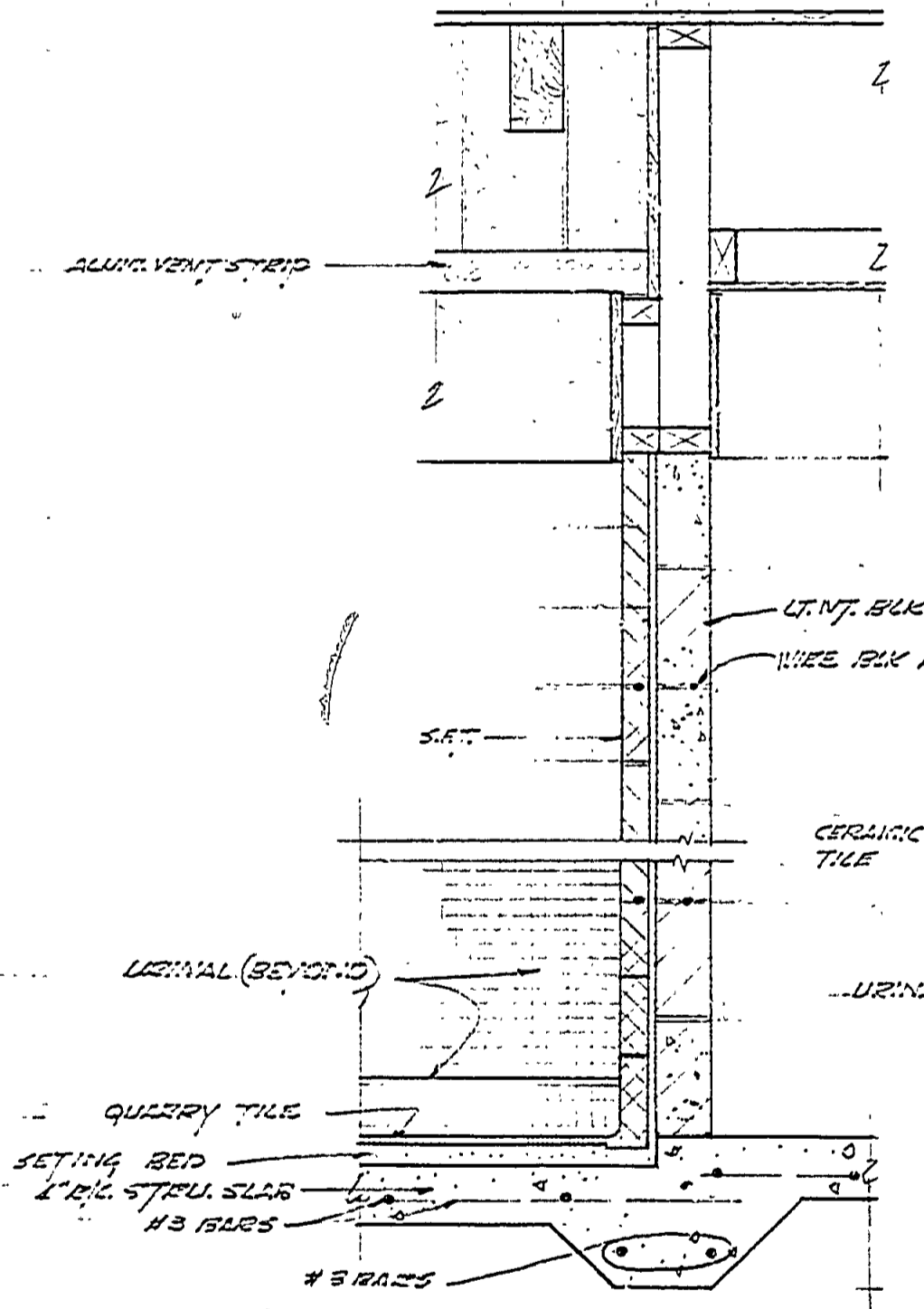
DET. 13 2/4
