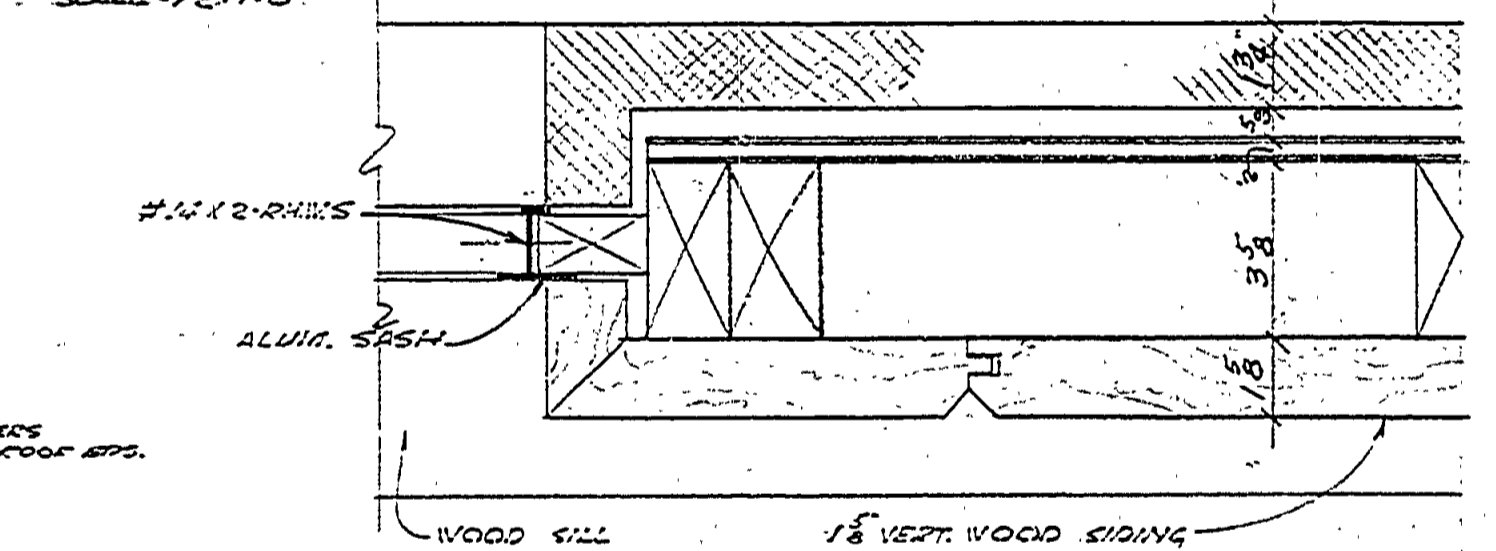
JAMB DET Scale 5/16\"/>
