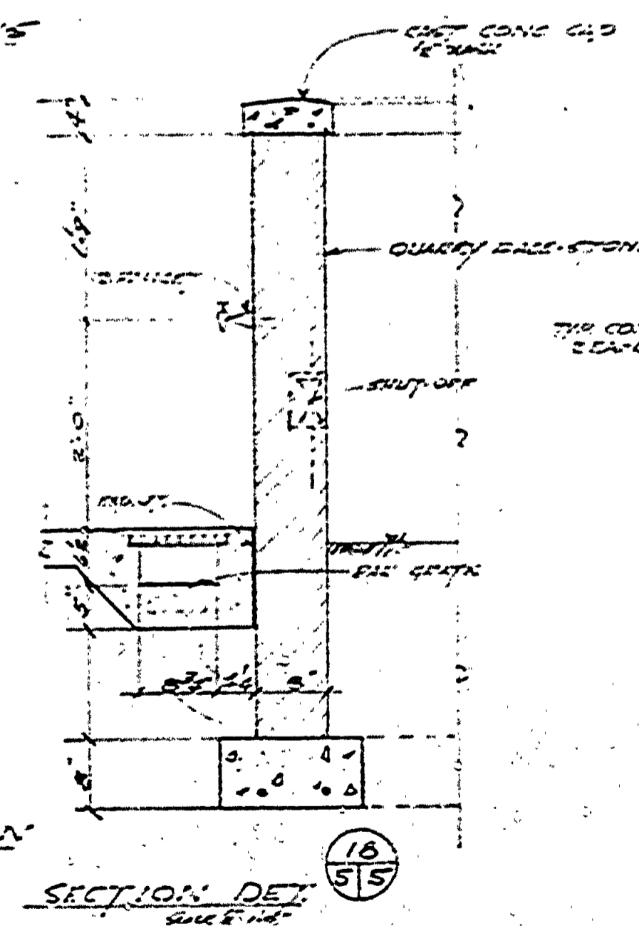
SECTION DET.
