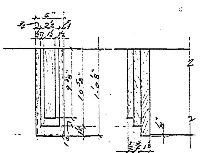
DET. END OF BOX BEAMS
