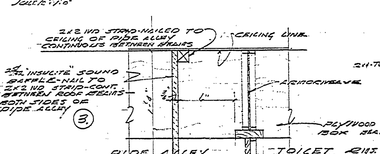
DET. "SOUND BAFLE"
