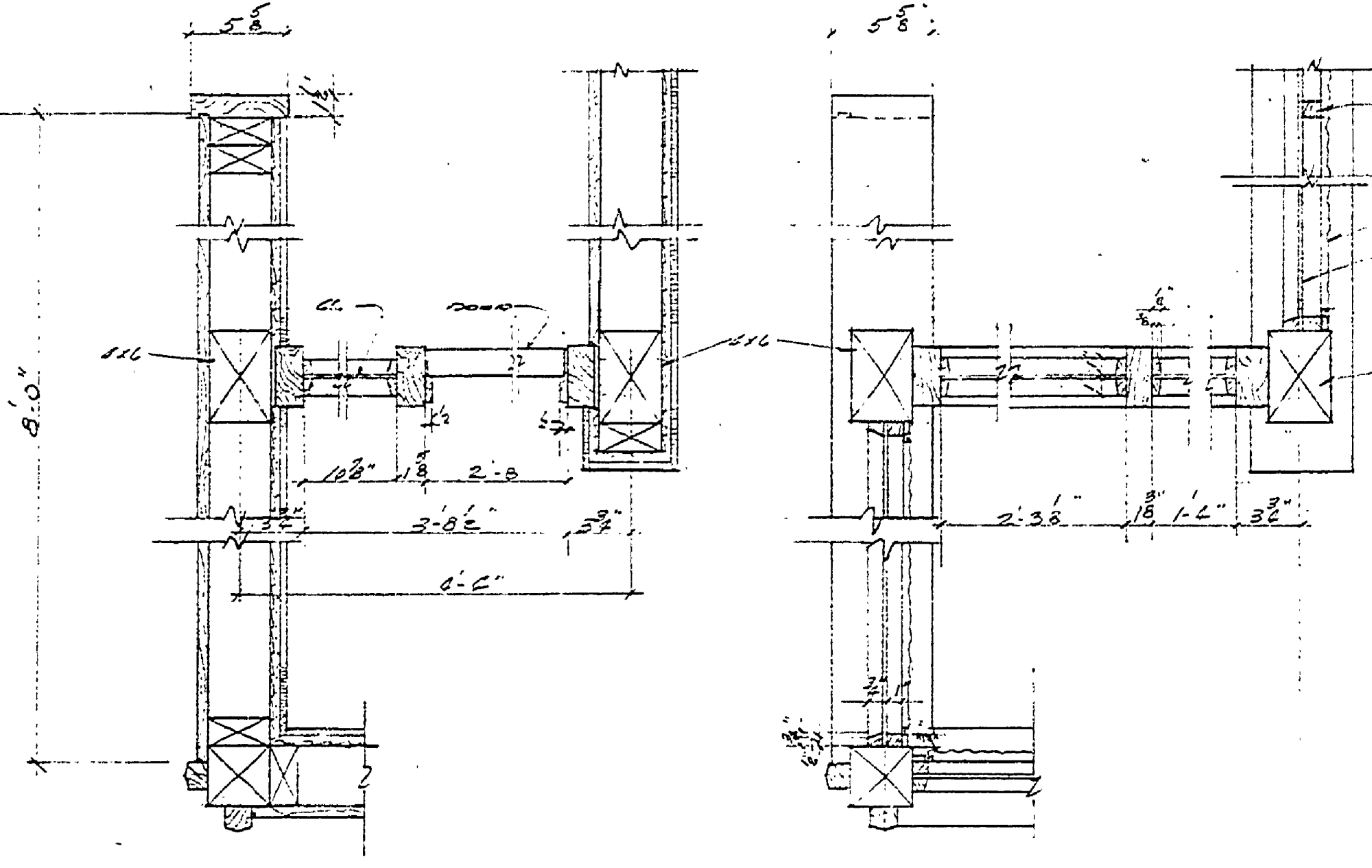
ENTRANCE DET.
