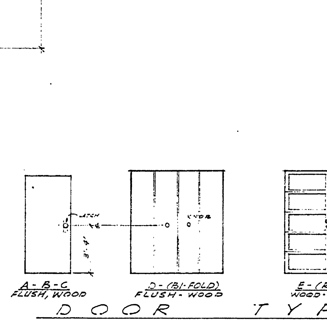
DOOR TYPES
