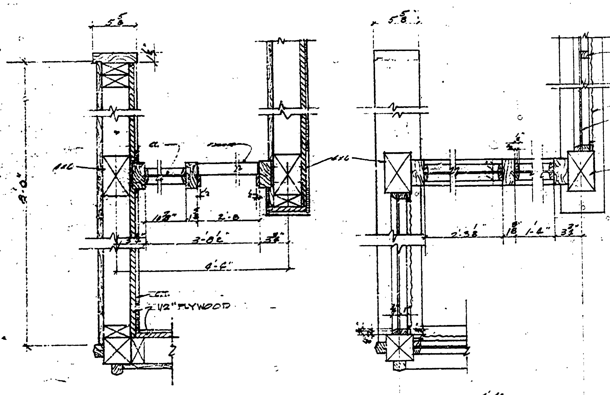
ENTRANCE DET. 9 SCALE: 1/8" = 1'-0"
