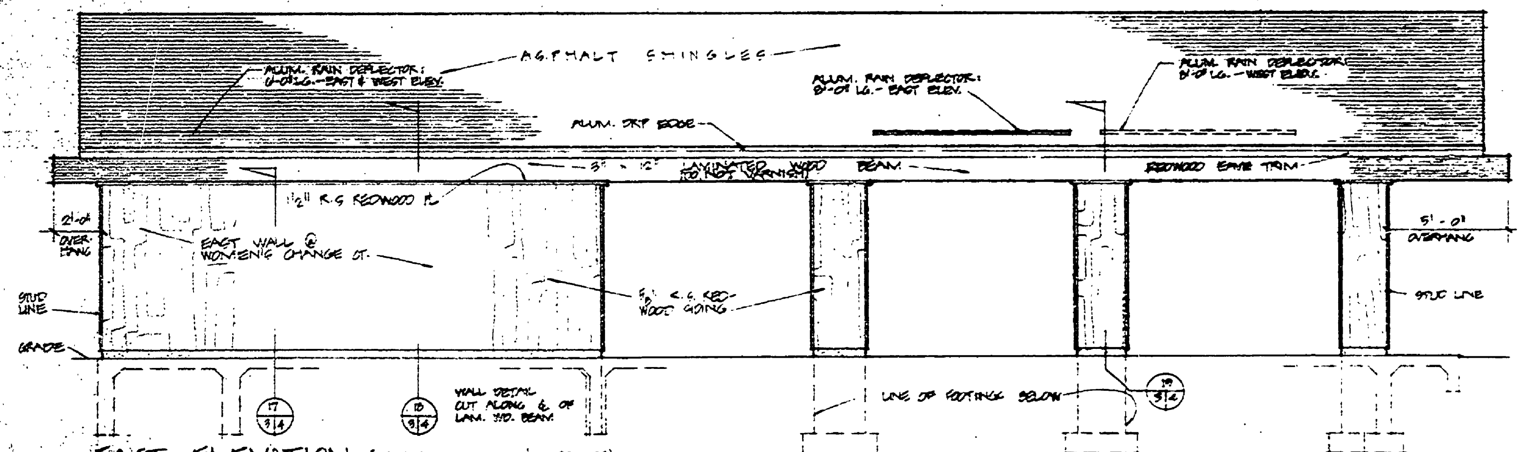
EAST ELEVATION (N. ELEV. SIMILAR & OPPOSITE) SCALE - 1/4" = ONE FOOT
