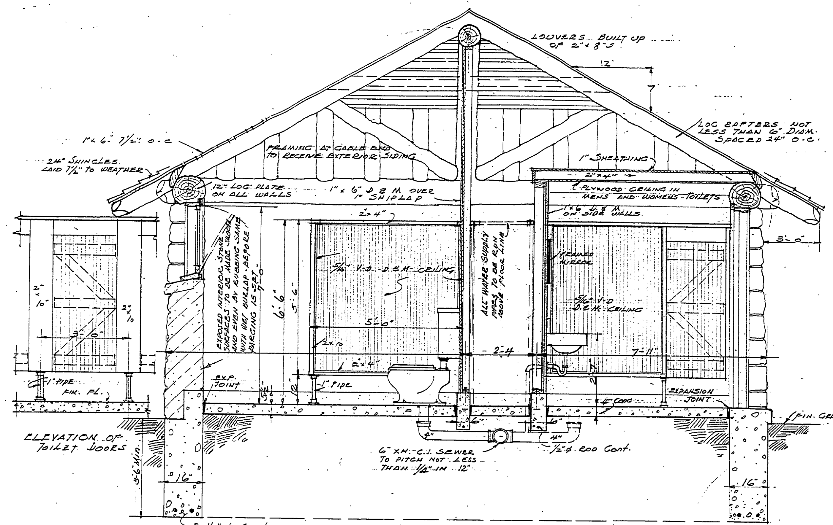
SECTION ON LINE A-A Scale: 1/2" = 1'-0"
