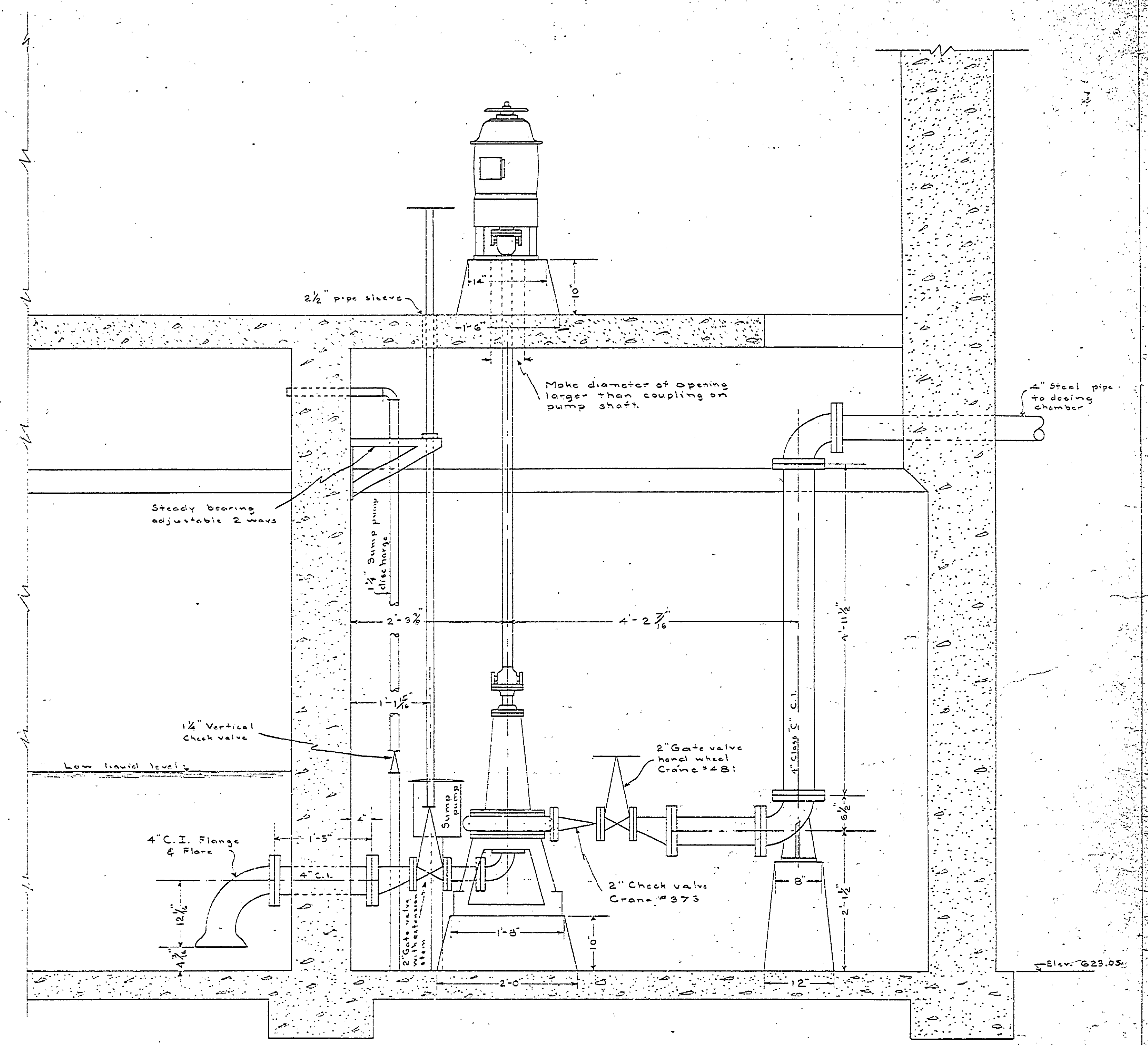
SECTION A-A SCALE: 1"=1'-0"
