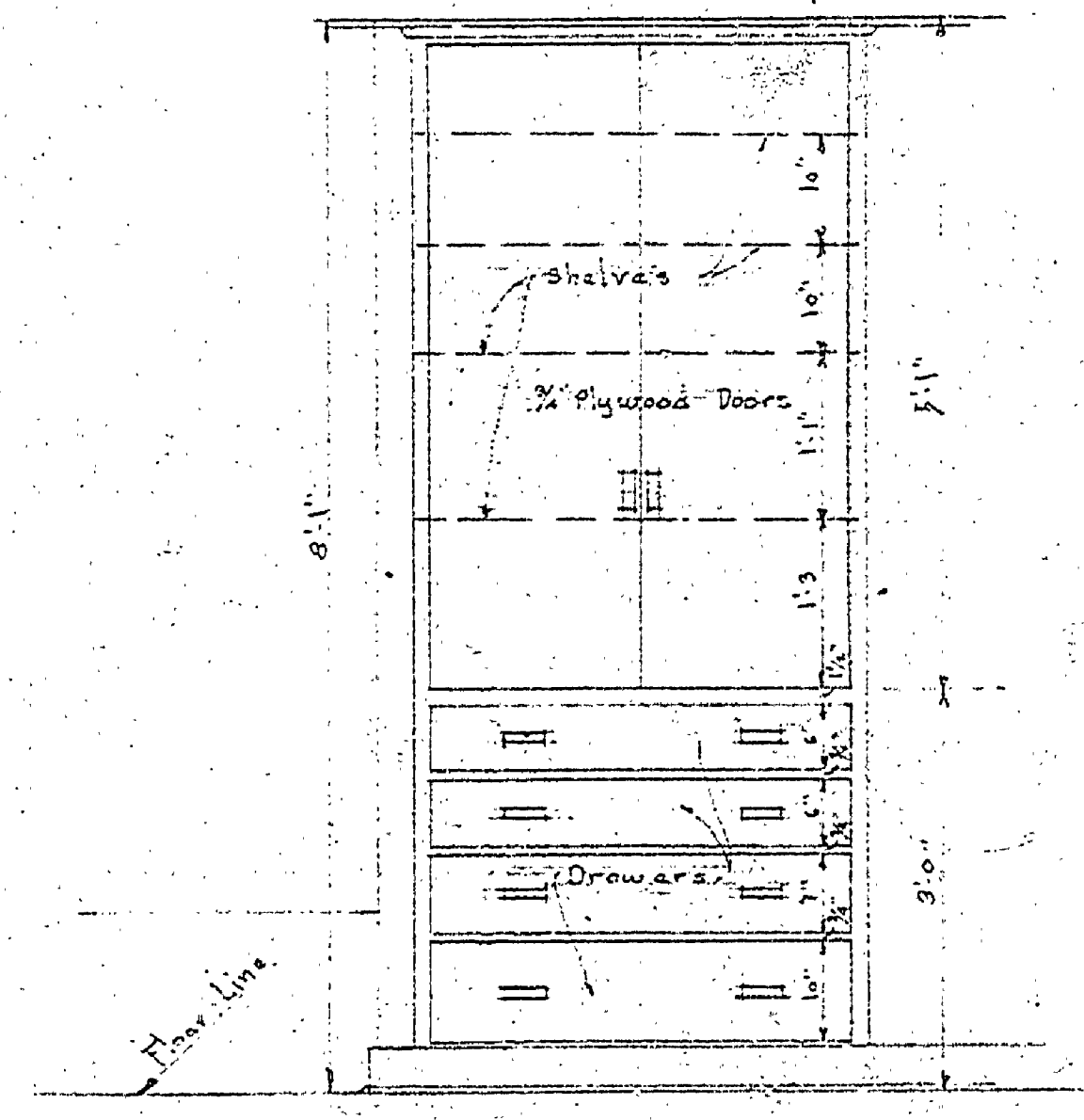
ELEVATION
