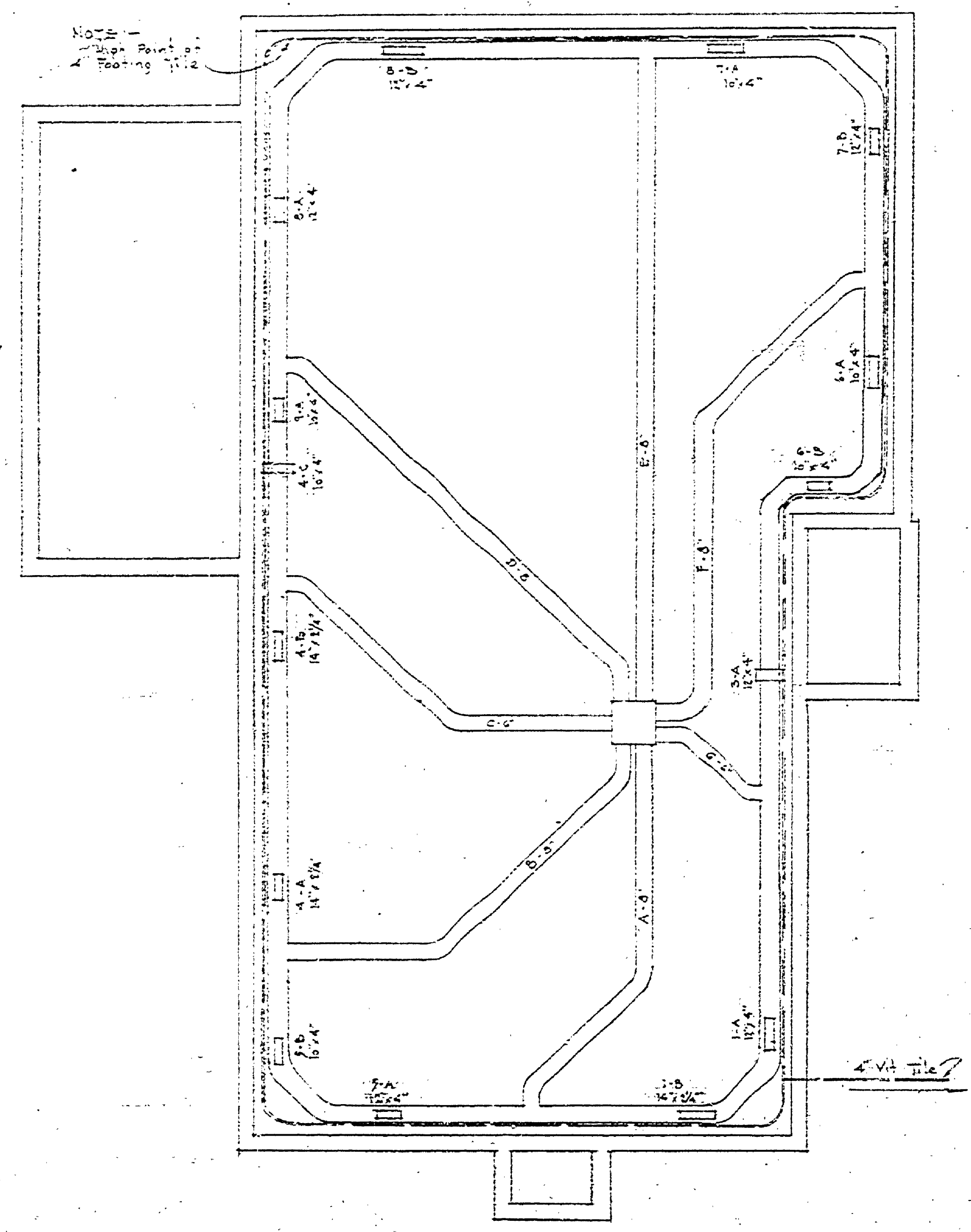
HEATING PLAN Scale: 1/8" = 1'-0"
