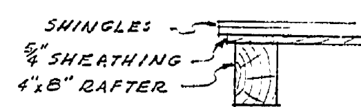
RAKE DETAIL SCALE: 1" = 1'-0"
