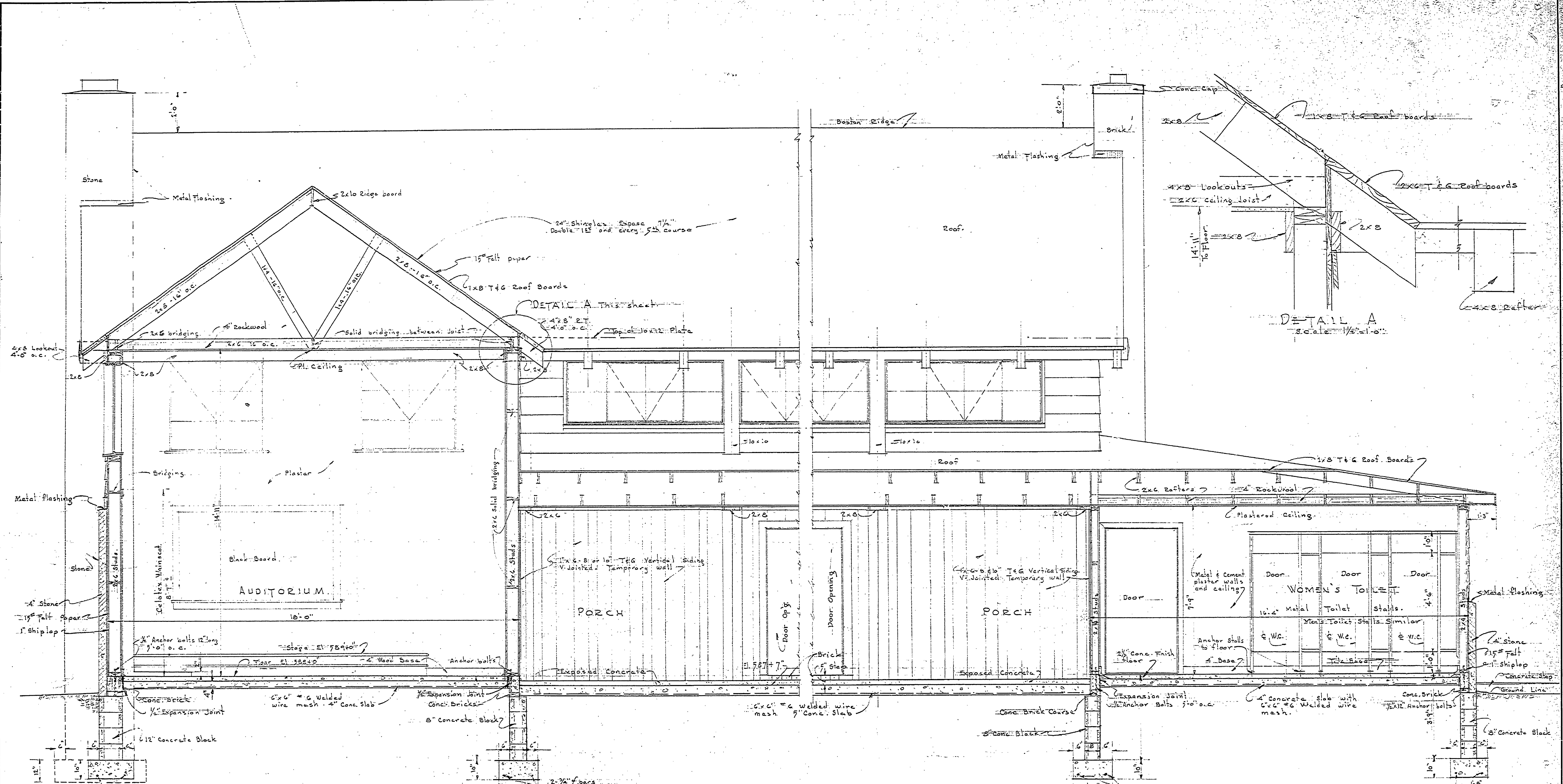
LONGITUDINAL SECTION A-A Scale: 1/4" = 1'-0"
