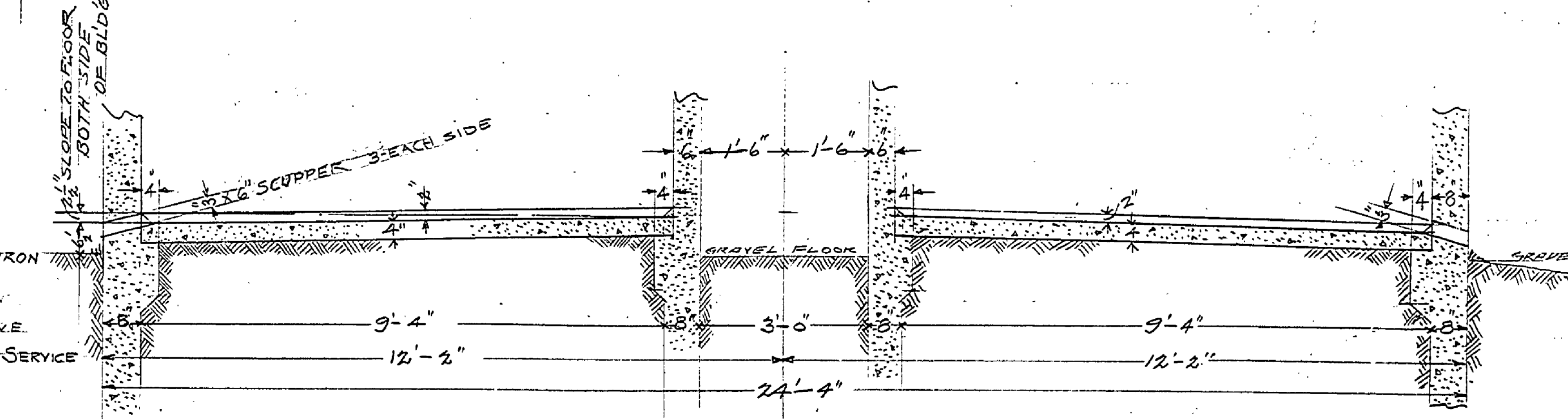
SECTION A-A
