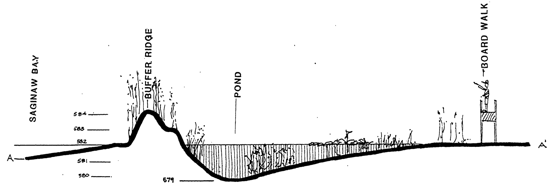
A-SECTION - A' SCALE: 1" = 30' (HORIZ.) 1" = 3' (VERT.)
